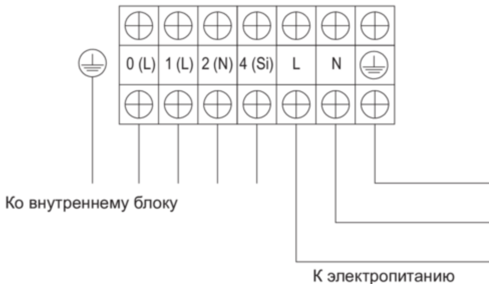
Клеммный терминал наружного блока
